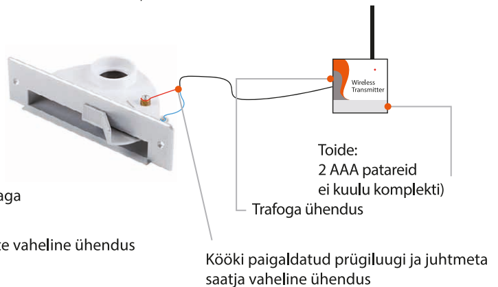
Juhtmeta saatja kööki paigaldatud prügiluugiga ühendamise skeem
